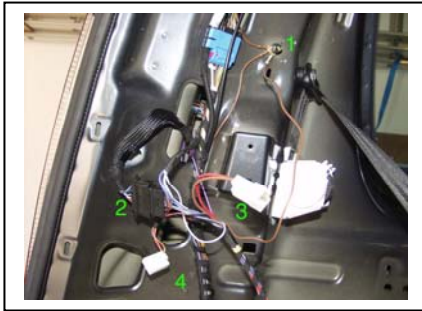
Steckverbinder D-Säule links
